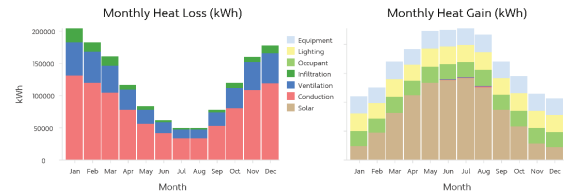
Energiebilanz - Sefaira
