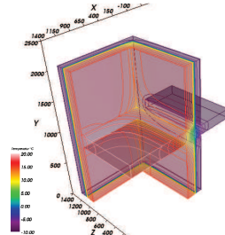
Wärmebrückenanalyse - Antherm
