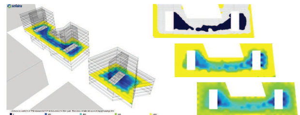
Tageslichtanalyse LUX - Sefaira
