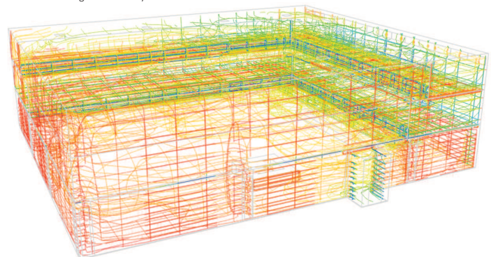
Tageslichtanalyse LUX - Sefaira
