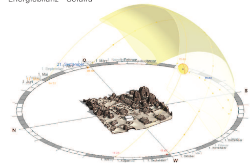
Verschattungsstudie - Revit
