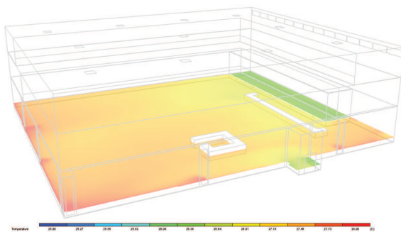
Temperaturverteilung - Design Builder
