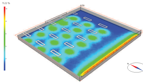
Tageslichtanalyse TLQ - IDA ICE
